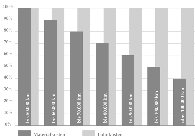
Materialkosten nach Betriebsleistung des beschädigten Bauteils
